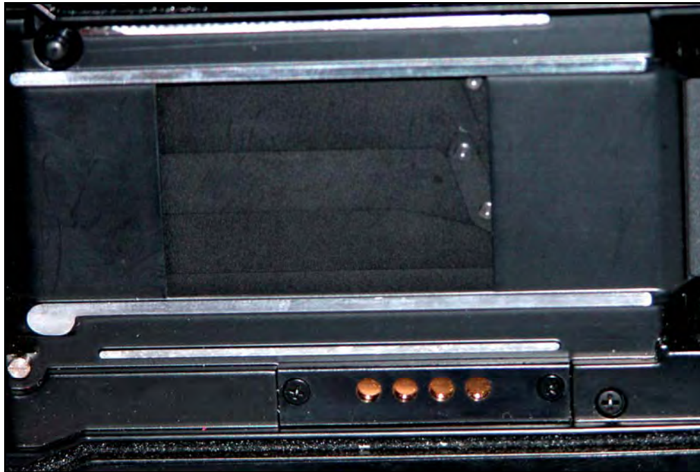
٤. الغالق (الشتري)
